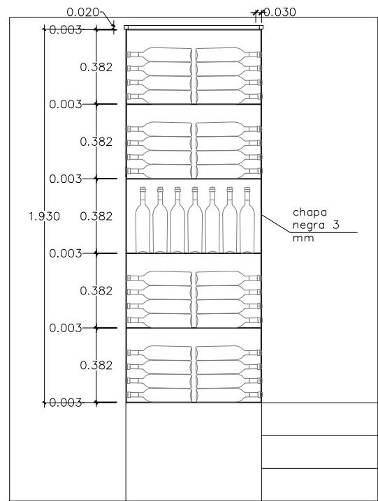
Corte Botellero cava vinos
