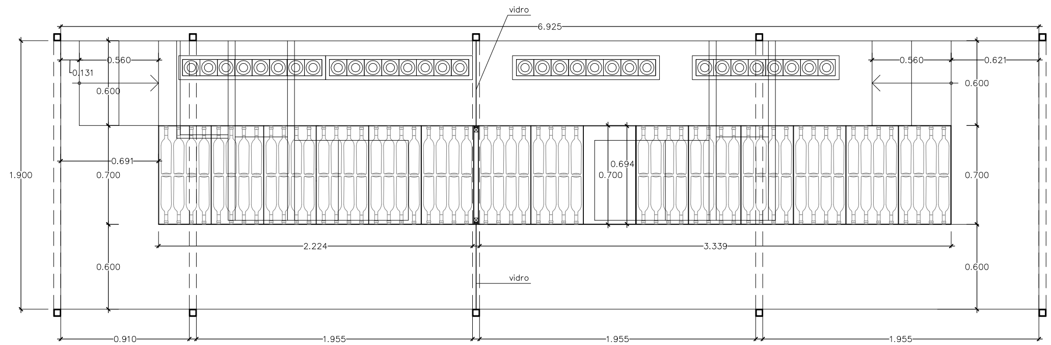
Planta interior tarima, para máquinas
