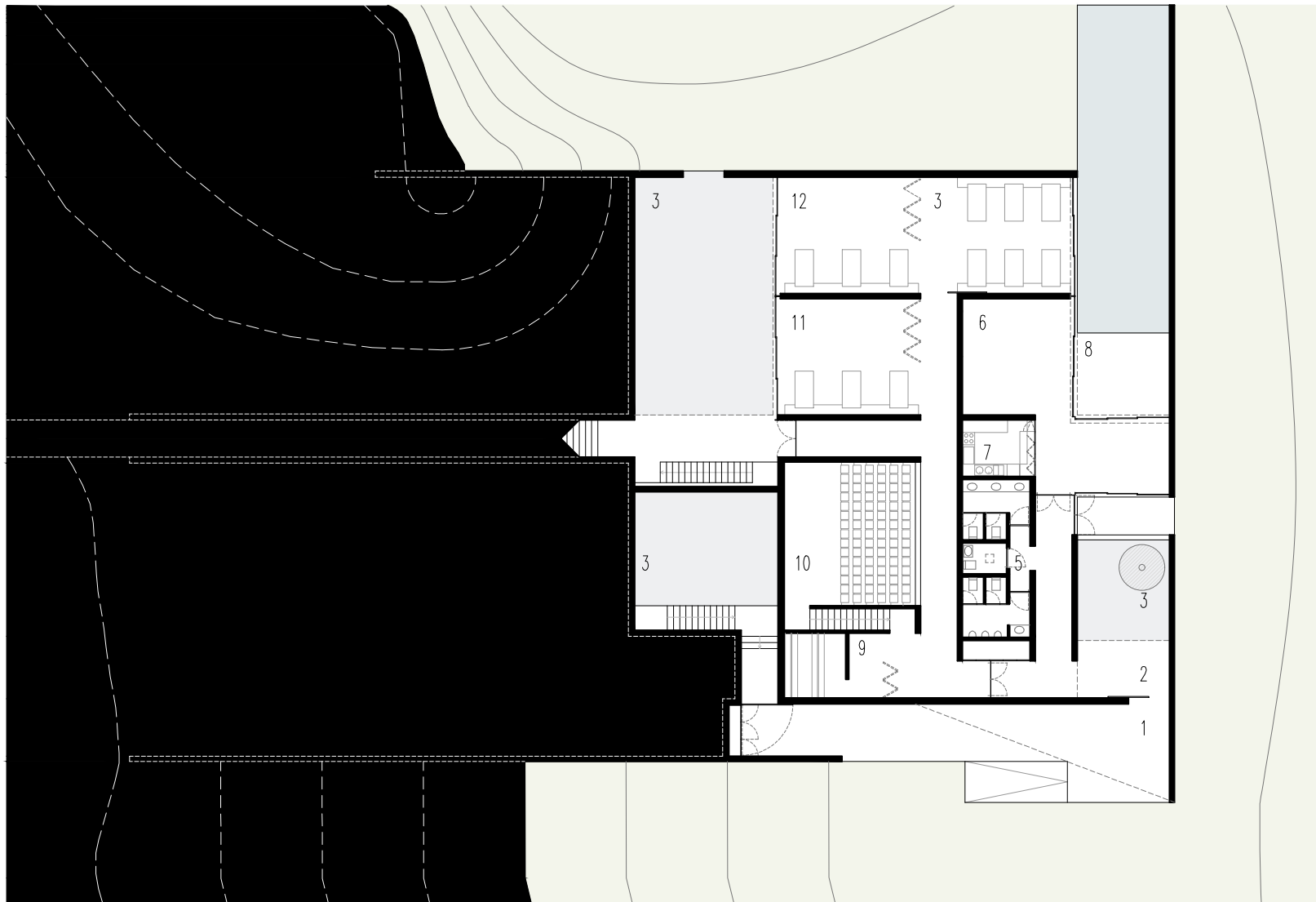
CENTRO DE EDUCAÇÃO AMBIENTAL - PLANTA DO PISO 0
