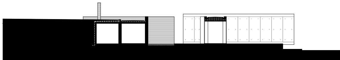
EDIFÍCIO DA EQUIPE DE GESTÃO DO PARQUE - PERFIL 3.3'
