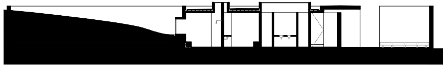
BALNEÁRIOS - PERFIL 1. 1'
