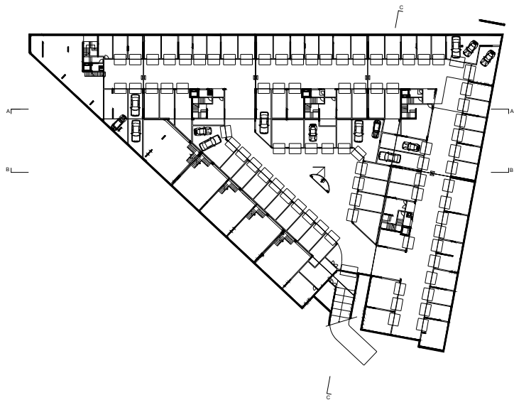
PLANTA PISO -1
