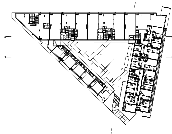
PLANTA PISO 0
