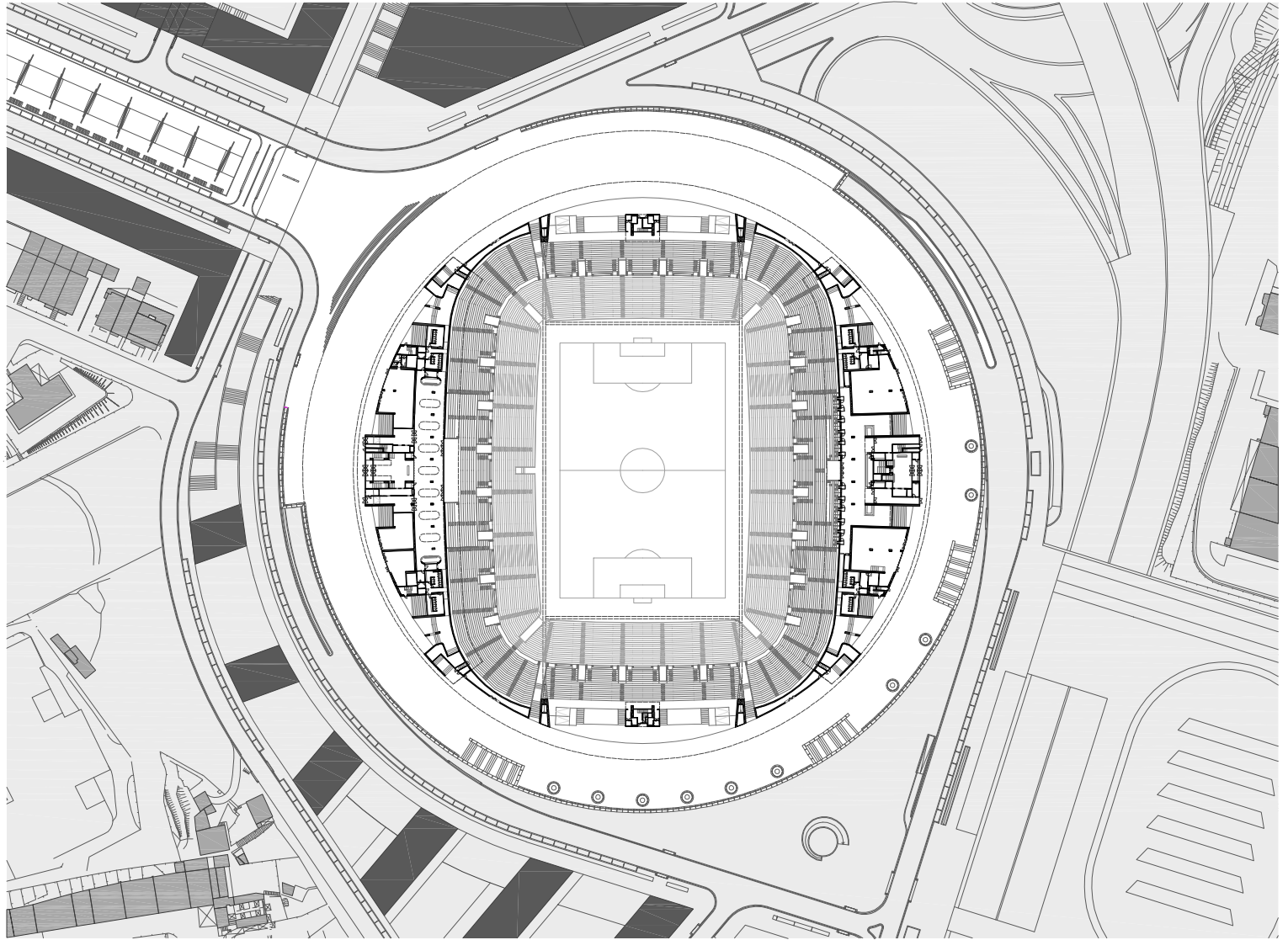
PLANTA DO PISO 0 - ACESSOS / ACCESS
