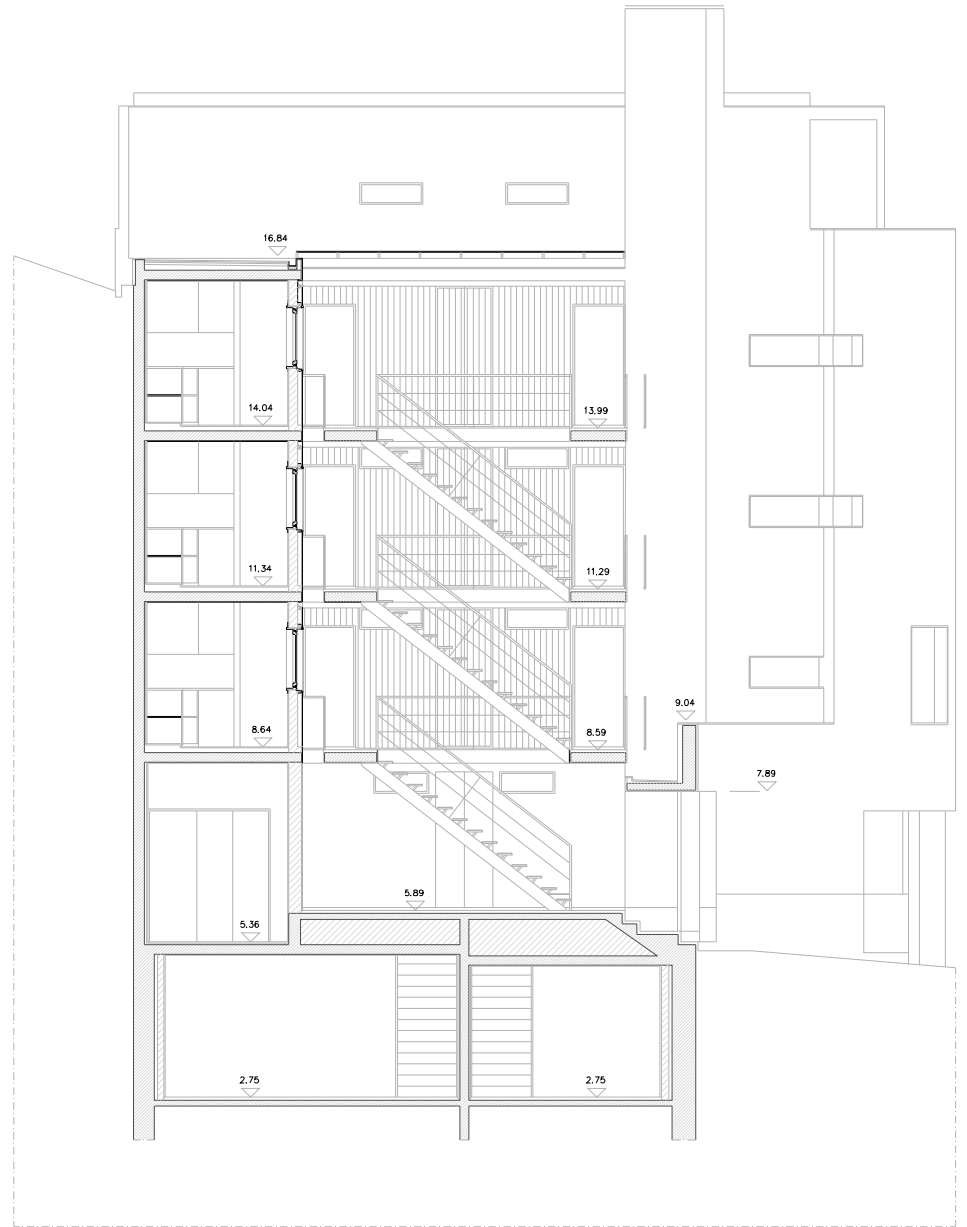
Corte AB
