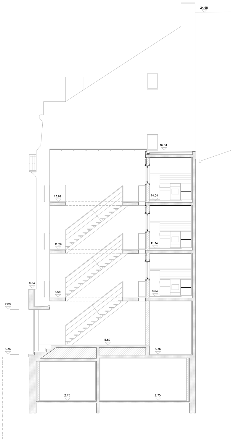
Corte EF
